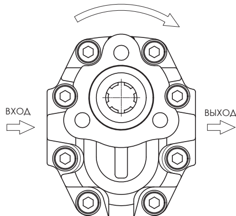
ВИД СПЕРЕДИ
